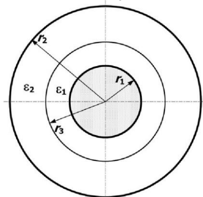
Рис. 2.9 – Кабель с градирированной изоляцией Радиус оболочки r_2 в этом случае может быть найден из равенства
