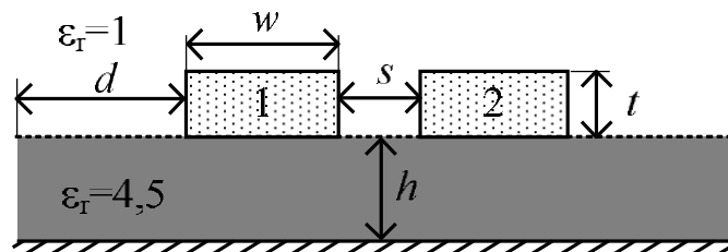
Рисунок 1.9 – Связанная линия и её параметры
