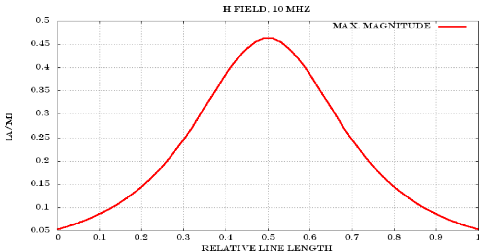
Рисунок 2.21 – График зависимости поля H от относительной длины линии
