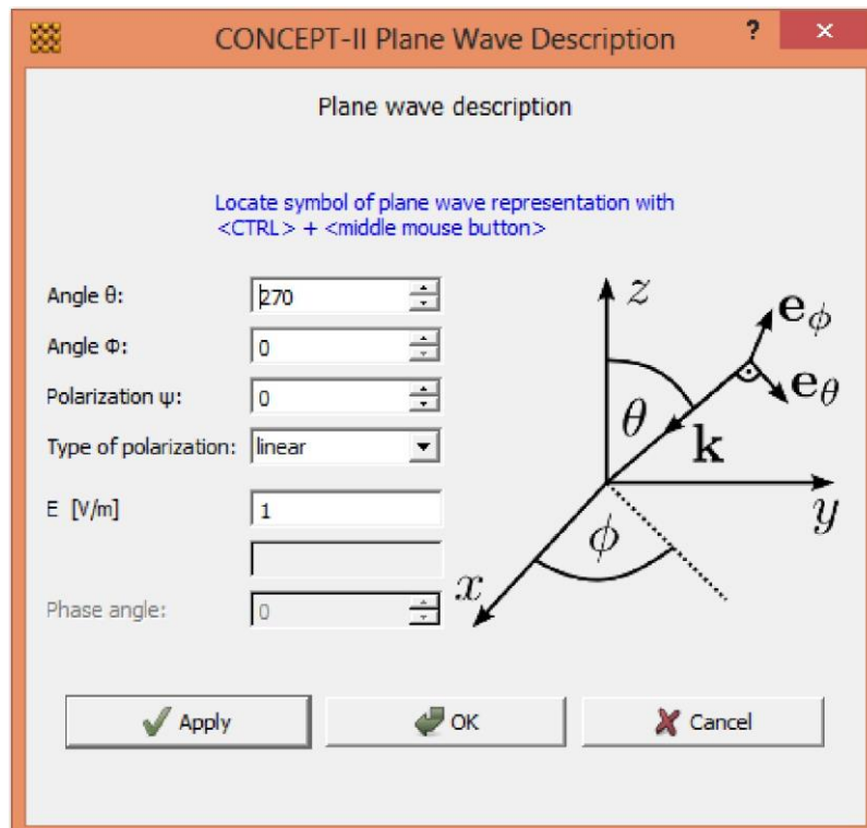
Рисунок 2.36 – Установка параметров поля плоской волны Для просмотра распределения тока на поверхности воспользоваться
