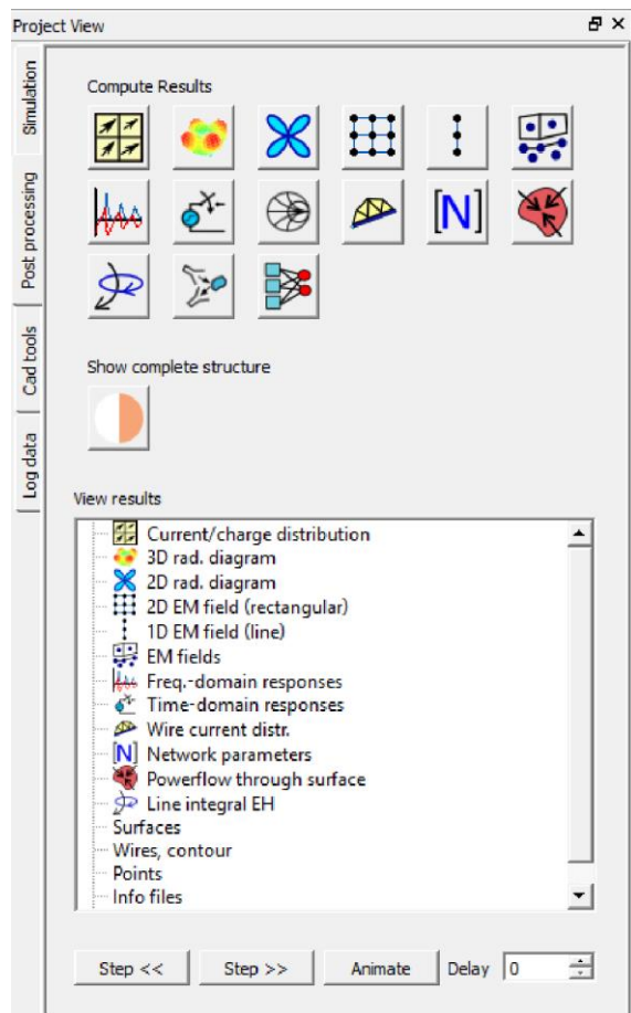
Рисунок 1.36 – Постобработка вычислений
