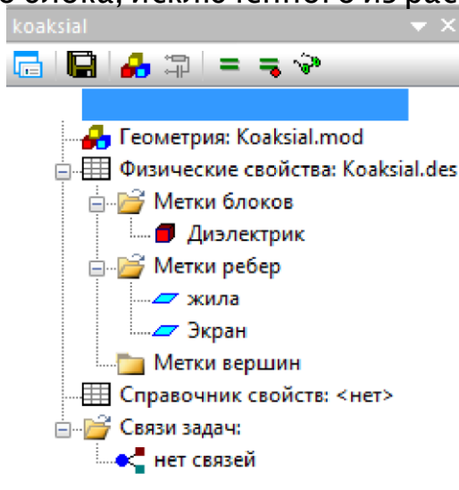
Рисунок 1.22 – Дерево задачи
