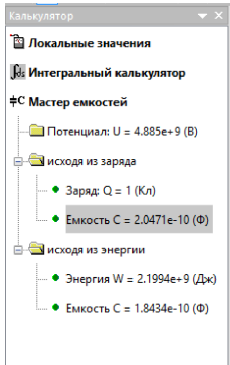
Рисунок 1.26 – Окно калькулятора
