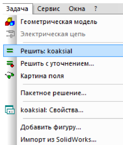
Рисунок 1.23 – Вкладка задача
