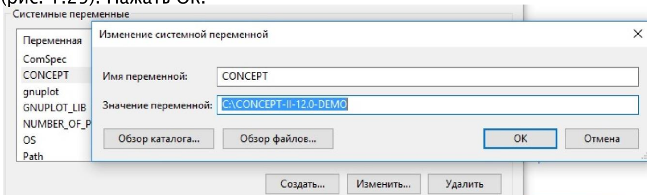
Рисунок 1.29 – Расширение пути
