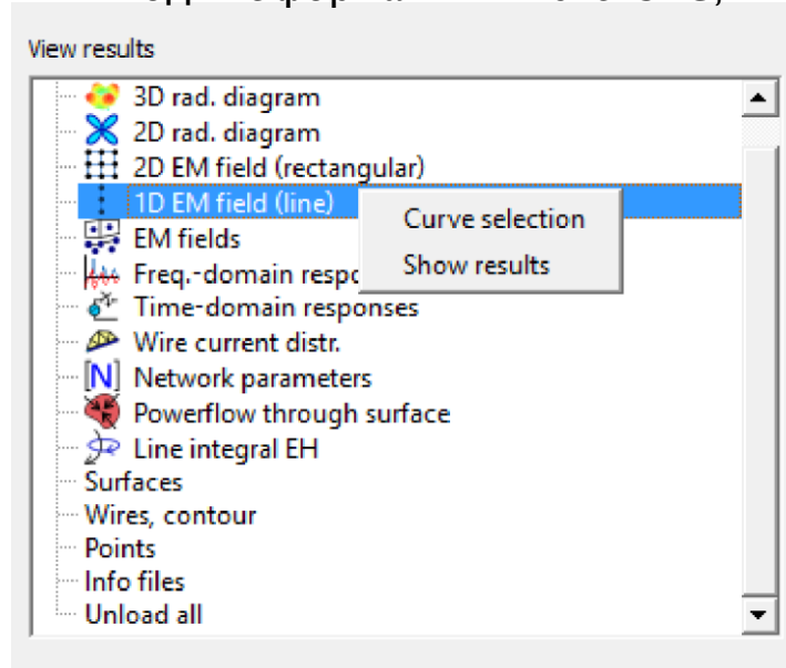
Рисунок 2.22 – Дерево пост-обработки
